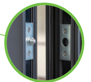
Pions de sécurité anti-dégondrage
