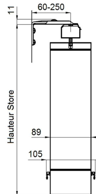
Détail rail supérieur
