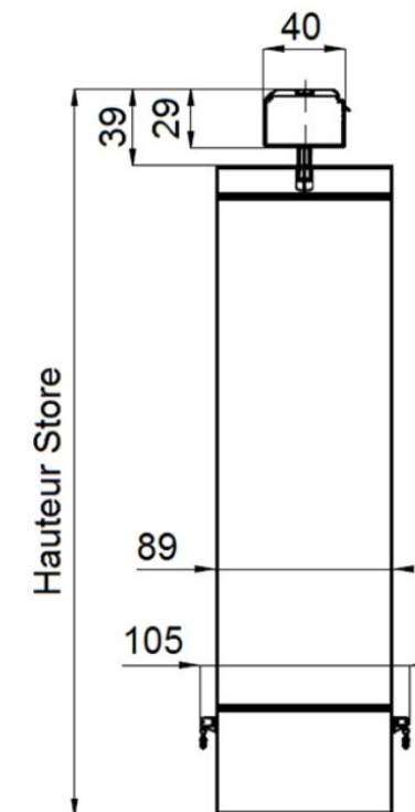
Détail rail supérieur
