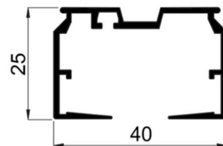
Détail rail supérieur
