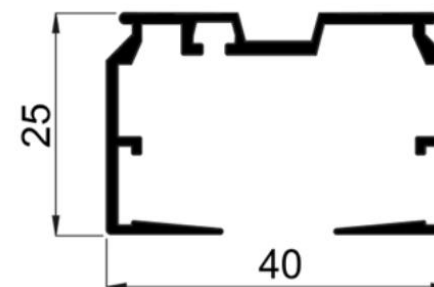
Détail rail supérieur
