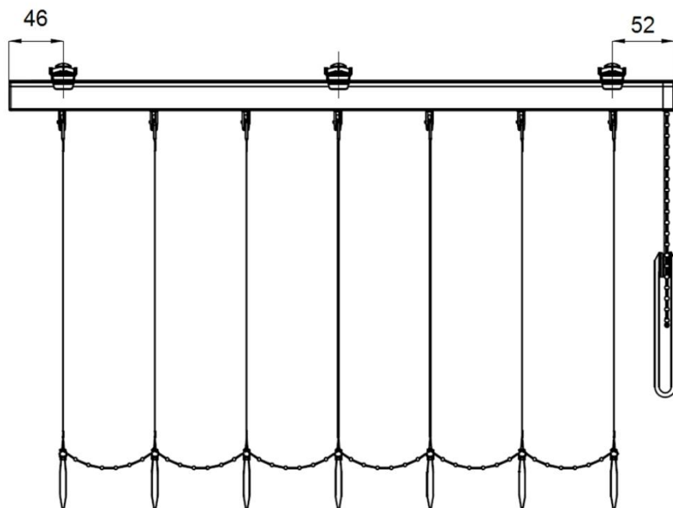
Vue de dessus pose de face
