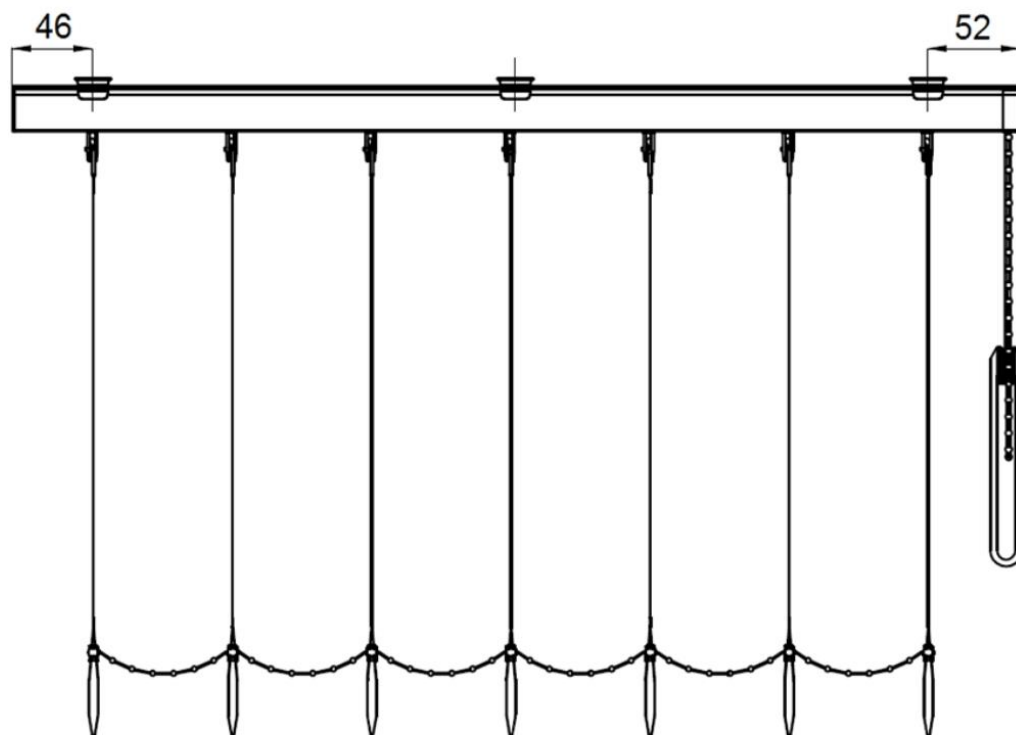
Vue de dessus pose plafond
