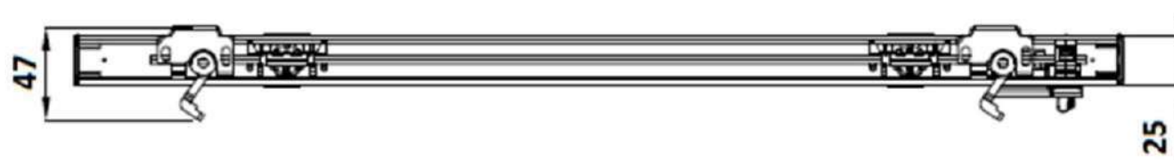
Vue de dessus - Pose de face
